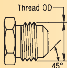
SAE 45° Flare Male (MS)
